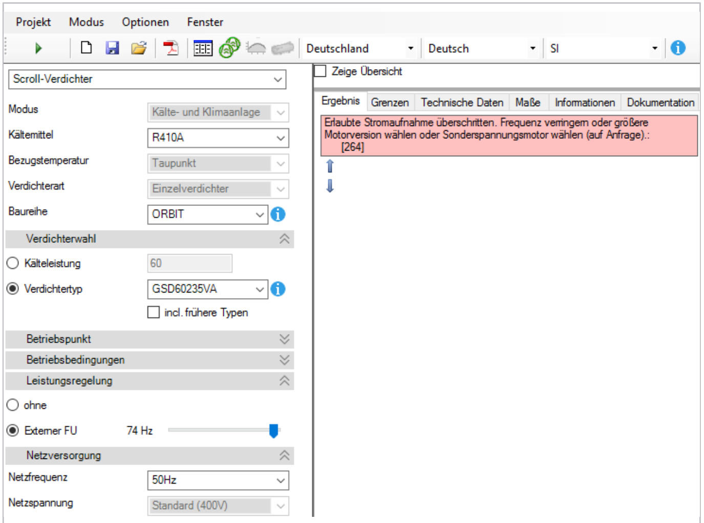
Abb. 6: Erhöht man die Betriebsfrequenz eines gewählten Verdichters, kann die maximale Stromaufnahme überschritten werden. Die Software empfiehlt dann z.B. einen Sonderspannungsmotor.
