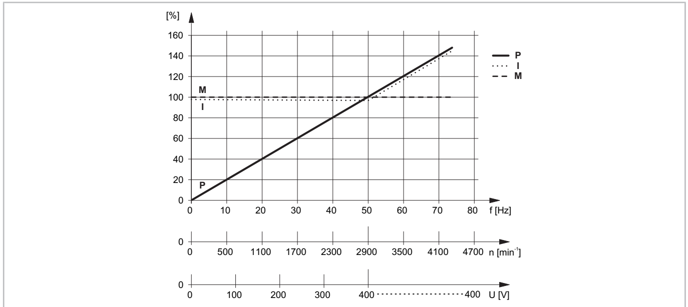
Abb. 3: Betriebscharakteristik eines ORBIT Verdichtermotors (E..7 Serie: max. 65 Hz) bei Betrieb mit Frequenzumrichter (400 V/3/50 Hz) mit Reserve.
