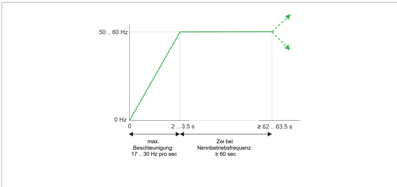
Abb. 16: Beispiel für eine Startsequenz für ORBIT und ESH7 Scrollverdichter mit Frequenzumrichter..
