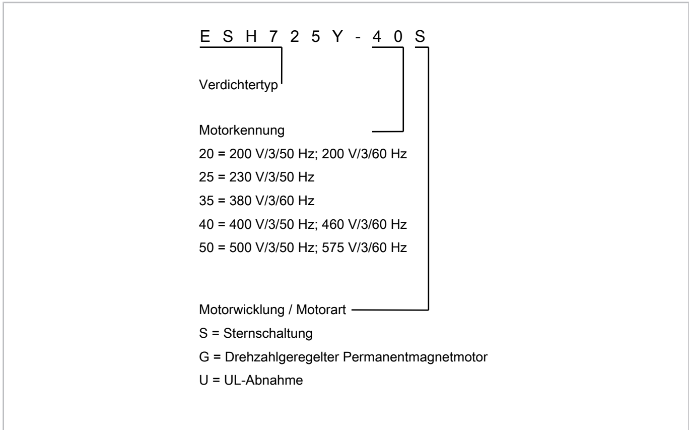
Abb. 11: Erläuterung der Motorerkennung bei Scrollverdichtern der Serien ESH7, ELH7, ELA7 (Beispiel hier: ESH7)
