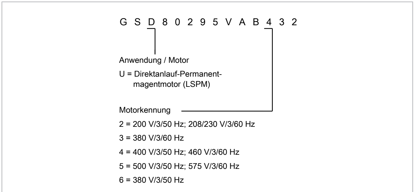
Abb. 10: Erläuterung der Motorkennung bei Scrollverdichtern der ORBIT Serie (Beispiel hier: GSD)
