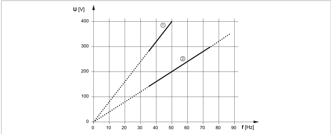
Abb. 14: Spannungsanstieg eines ORBIT Verdichtermotors (E..7 Serie: max. 65 Hz) über der Frequenz bei verschiedenen Motoren
