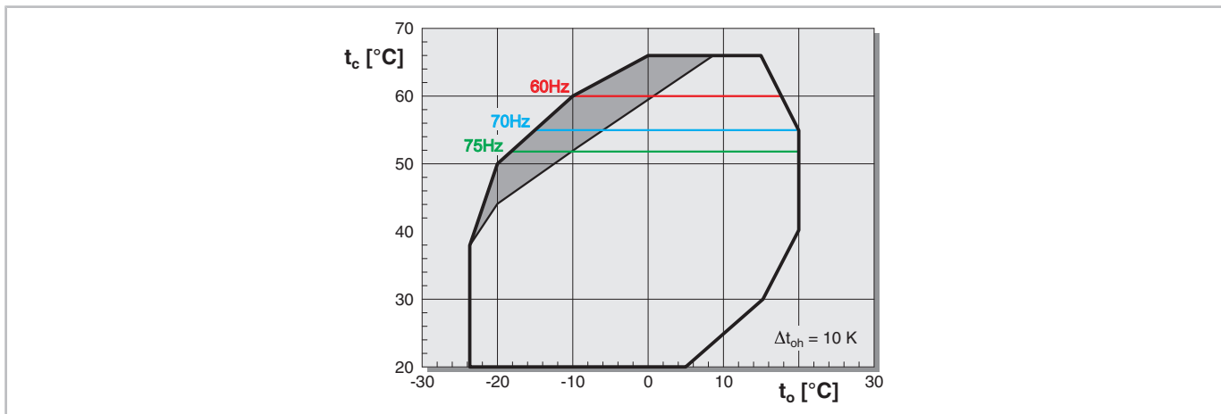
Abb. 4: Vereinfachtes Beispiel für Einsatzgrenzen eines ORBIT Scrollverdichters mit Frequenzumrichter bei 60, 70 und 75 Hz (Beschränkungen durch die Motortemperatur oder maximale Stromstärke). Der Verdichter darf nur im Bereich unterhalb der Frequenzlinien betrieben werden.
