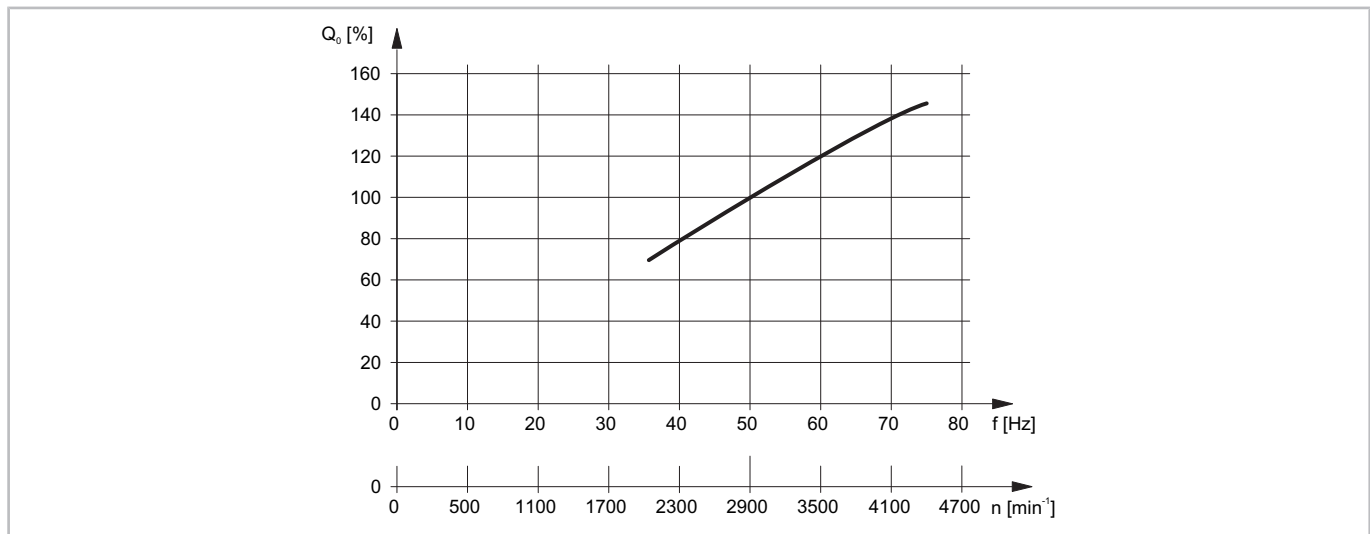
Abb. 2: Typischer Verlauf der Kälteleistung Q_0 in Abhängigkeit von Drehzahl und Frequenz bei einem ORBIT Verdichter (E..7 Serie: max. 65 Hz)
