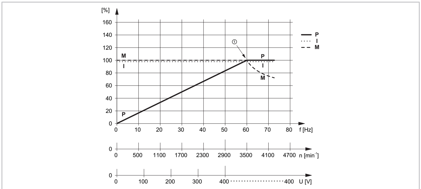
Abb. 13: Betriebscharakteristik eines ORBIT Verdichtermotors (E..7 Serie: max. 65 Hz) bei Betrieb mit Frequenzumrichter (380 V/3/60 Hz) ohne Reserve (Strom/Leistung), d.h. Motor am Betriebspunkt mit maximaler Leistung.
