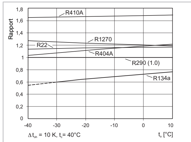
Fig. 3: Puissance frigorifique volumétrique de différents fluides frigorigères par rapport à R290 avec un débit de gaz d'aspiration identique
