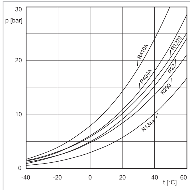
Fig. 2: Courbes de pression de vapeur de R290 et R1270 par rapport à R22 et aux fluides frigorigères HFC
